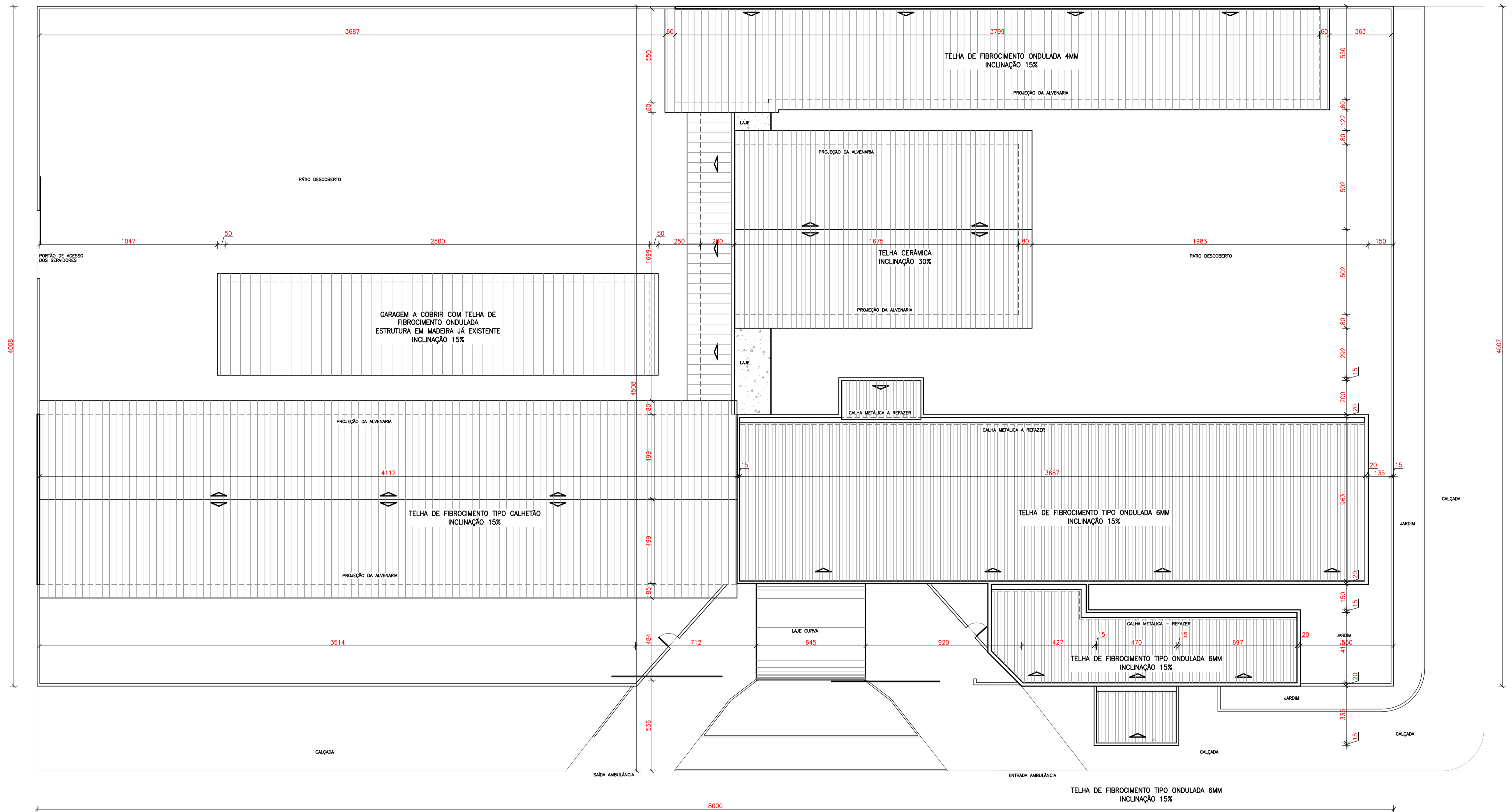
PLANTA DE COBERTURA ESCALA 1:75
